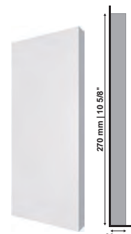
Sócalo 182 Plinth Block | Zócalin 110 x 270 x 20mm 4 5/16" x 10 5/8" x 13/16" Cód. | Code - 24342
