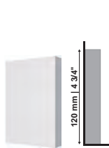
Sócalo 178 Plinth Block | Zócalin 80 x 120 x 20mm 3 1/8" x 4 3/4" x 13/16" Cód. | Code - 22396
