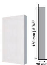
Sócalo 183 Plinth Block | Zócalin 70 x 150 x 20mm 2 3/4" x 5 7/8" x 13/16" Cód. | Code - 24343
