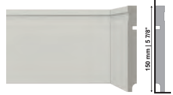
480 Rodapé Fendi Fendi Wall Base Zócalo Fendi
