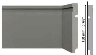
480 Rodapé Cinza Titanium Titanium Gray Wall Base Zócalo Gris Titanio
