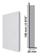
Sócalo 186 Plinth Block | Zócalin 80 x 160 x 20mm 3 1/8" x 6 5/16" x 13/16" Cód. | Code - 25361
